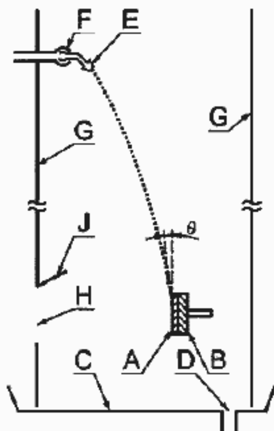
A – проба; B – держатель; C – поддон; D – сточное отверстие; E – струйное сопло; F – шарнирное соединение; G – корпус; H – квадратное отверстие; J – желоб
